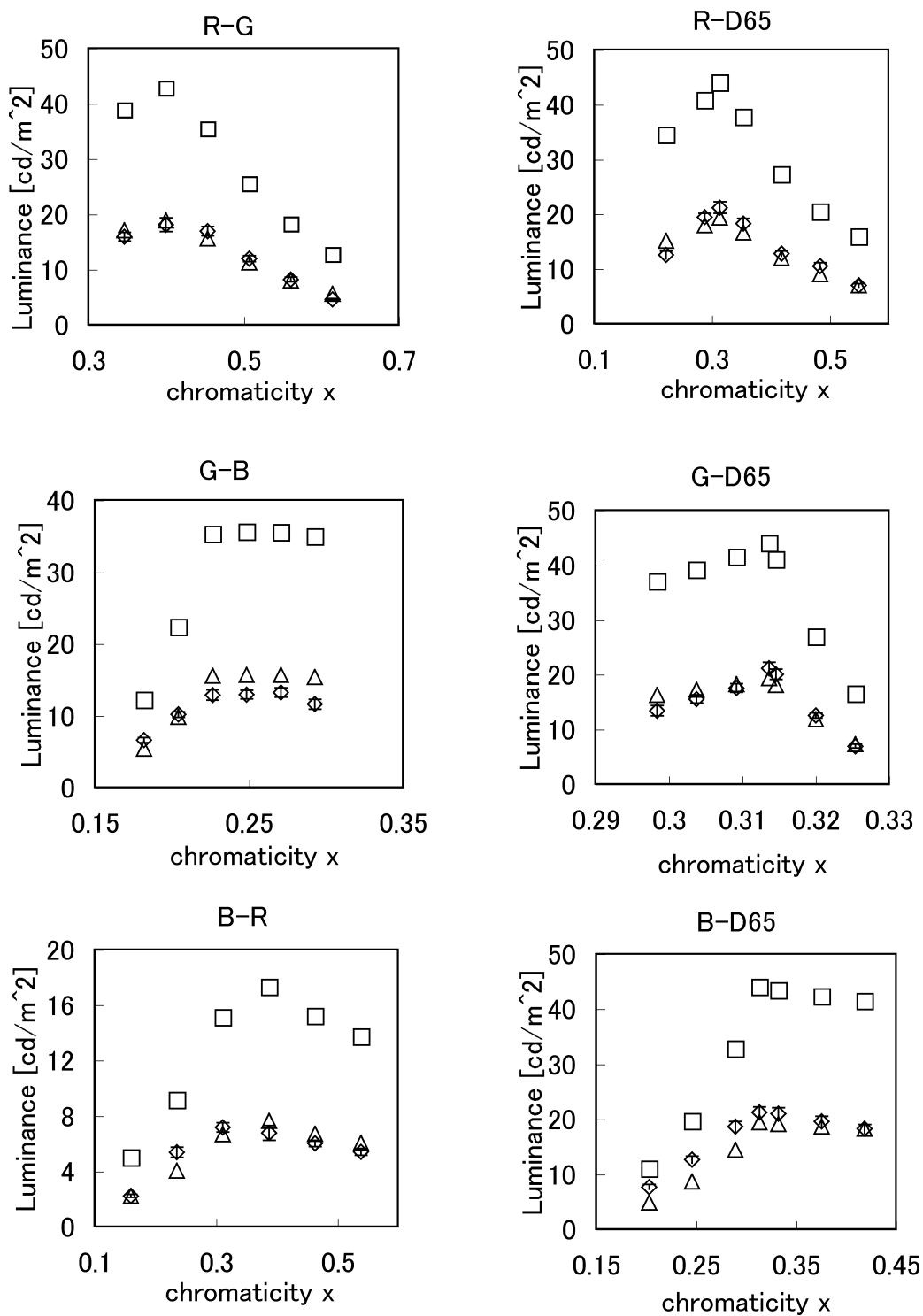
図3 被験者TFのモードの移行輝度 (○), オプティマルカラーの輝度 (□), オプティマルカラーの輝度と係数Cとの積 (△). R-D65の左から3個目の結果, G-D65の左から4個目の結果, B-D65の左から4個目の結果はすべてテスト刺激の色度がD65の色度であったときの結果を表す (つまり3個の点が1個の結果を表している).
