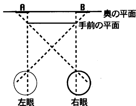
図1 半遮蔽部分。手前の平面が奥の平面を遮蔽しているとき、奥の平面に左右どちらか一方の目にしか見えない部分ができる。奥の平面のAの部分には左眼だけに見える、Bの部分は右眼だけに見える。
